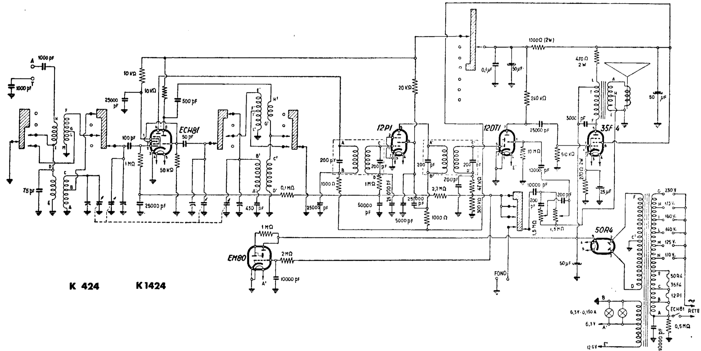
MAGNADYNE RADIO - Mod. A 24, K 424, K 1424 e S 124. Apparecchio a una gamma onde medie e tre gamme onde corte. Media frequenza a 471 kc/s. Potenza d'uscita 4 watt.
